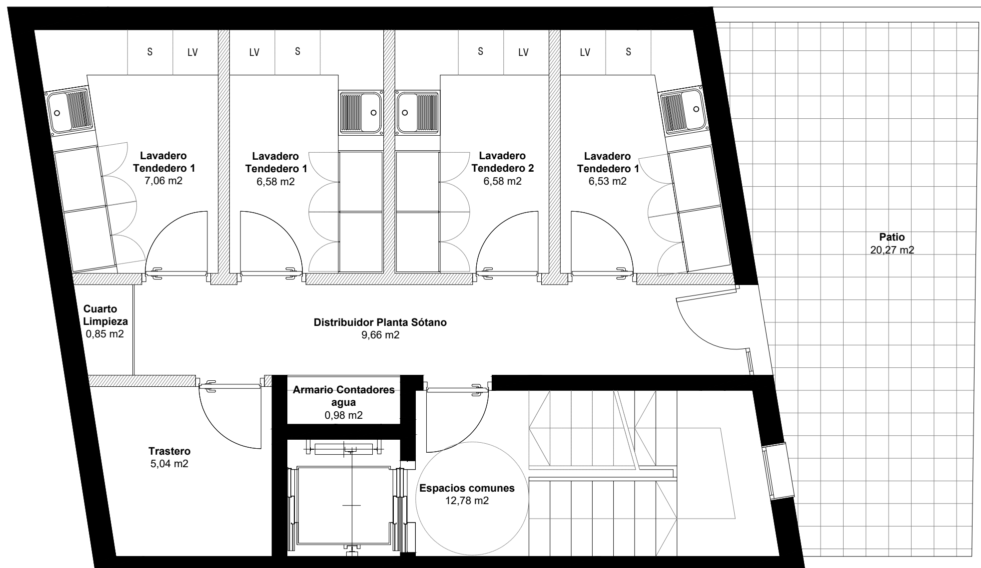
PLANTA SÓTANO
